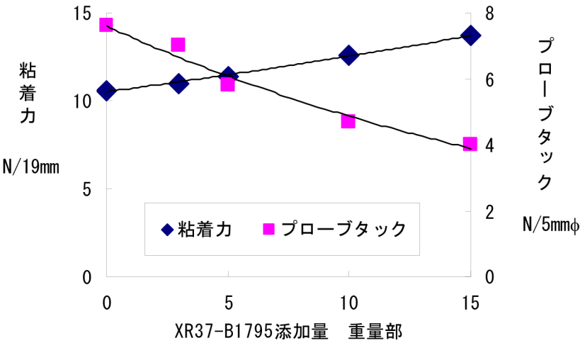
XR37-B1795添加によるXR37-B6722（過酸化物硬化型）の特性変化
